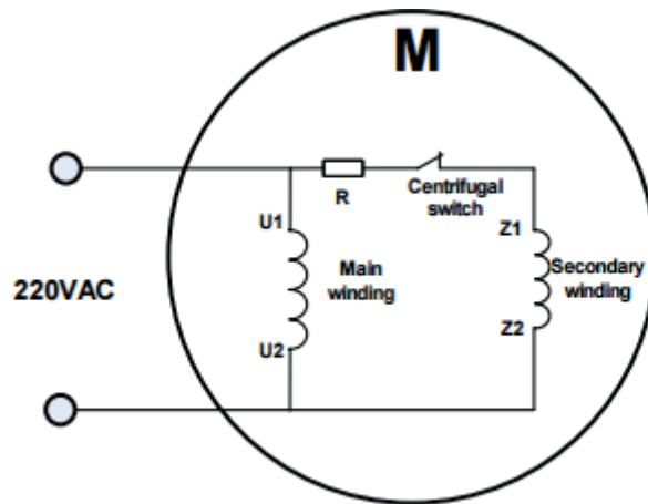
Şekil 2-9 Direnç başlatma modu: Motorun dahili kabloları
