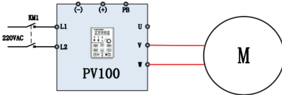
Şekil 2-15 PV100 ve motor arasındaki kablolama
