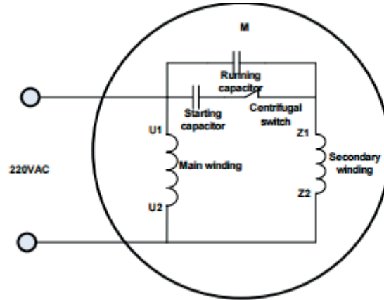
Şekil 2-8 Çift kondansatörlü motorun dahili kabloları
