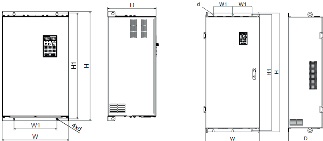
Şekil 1-4 18.5~30kW duvar montaj şeması
