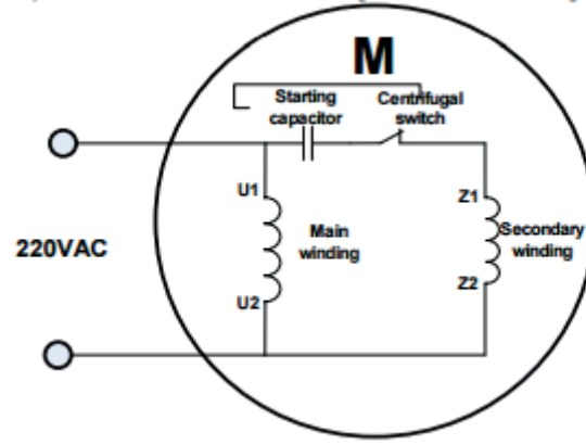
Şekil 2-7 Başlatma modu: Tek kondansatörlü motorun dahili kabloları
