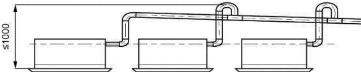
T-mafsalsız yakınsama tahliye boruları
