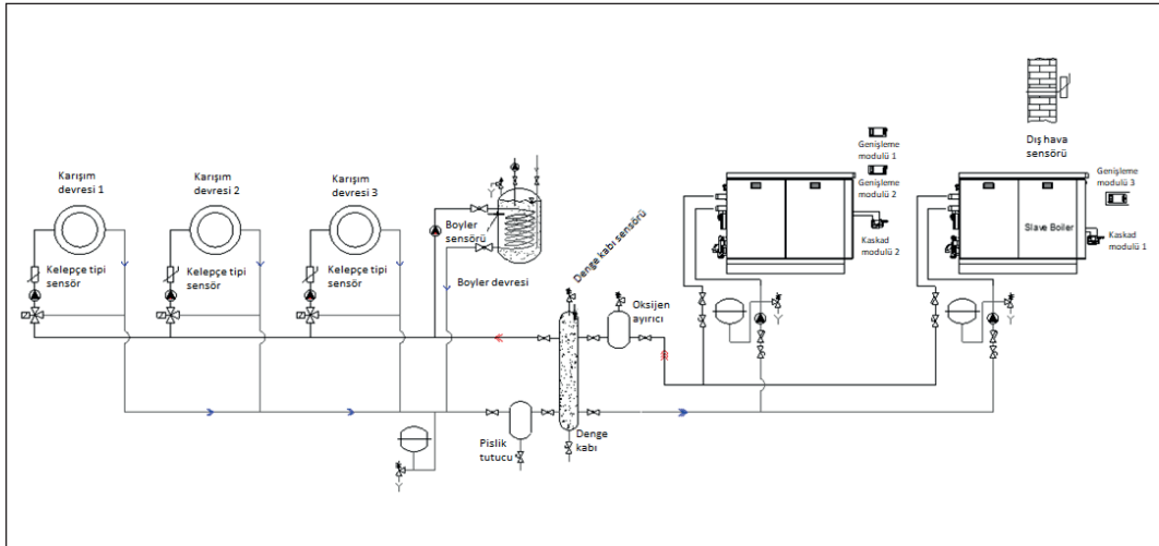
İki (kaskad çalışan) kazan, 3 karışım devresi, 1 boiler devresi bağlantı örneği (denge kabı ile)
