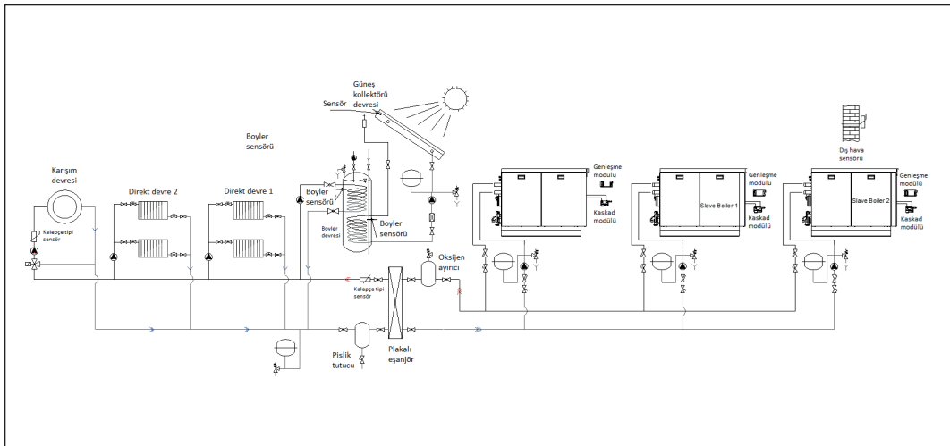
Üç (kaskad çalışan) kazan, 2 direkt devre, 1 karışım devresi, 1 güneş kolektörlü boiler devresinin primer ve sekonder devreyi ayırıcı plakalı eşanjör ile bağlantı örneği
