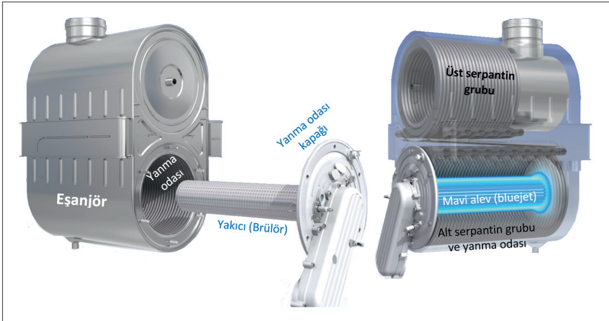
A. Aldens F-175, F-200, F-235, F-265 tipi eşanjör
